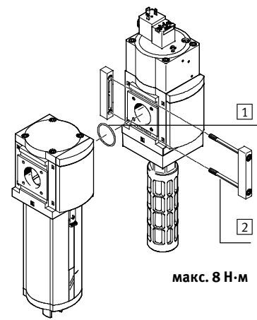
Fig. 6 Сборка
