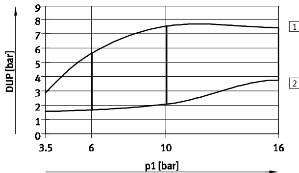
Fig. 13 Точка переключения давления
